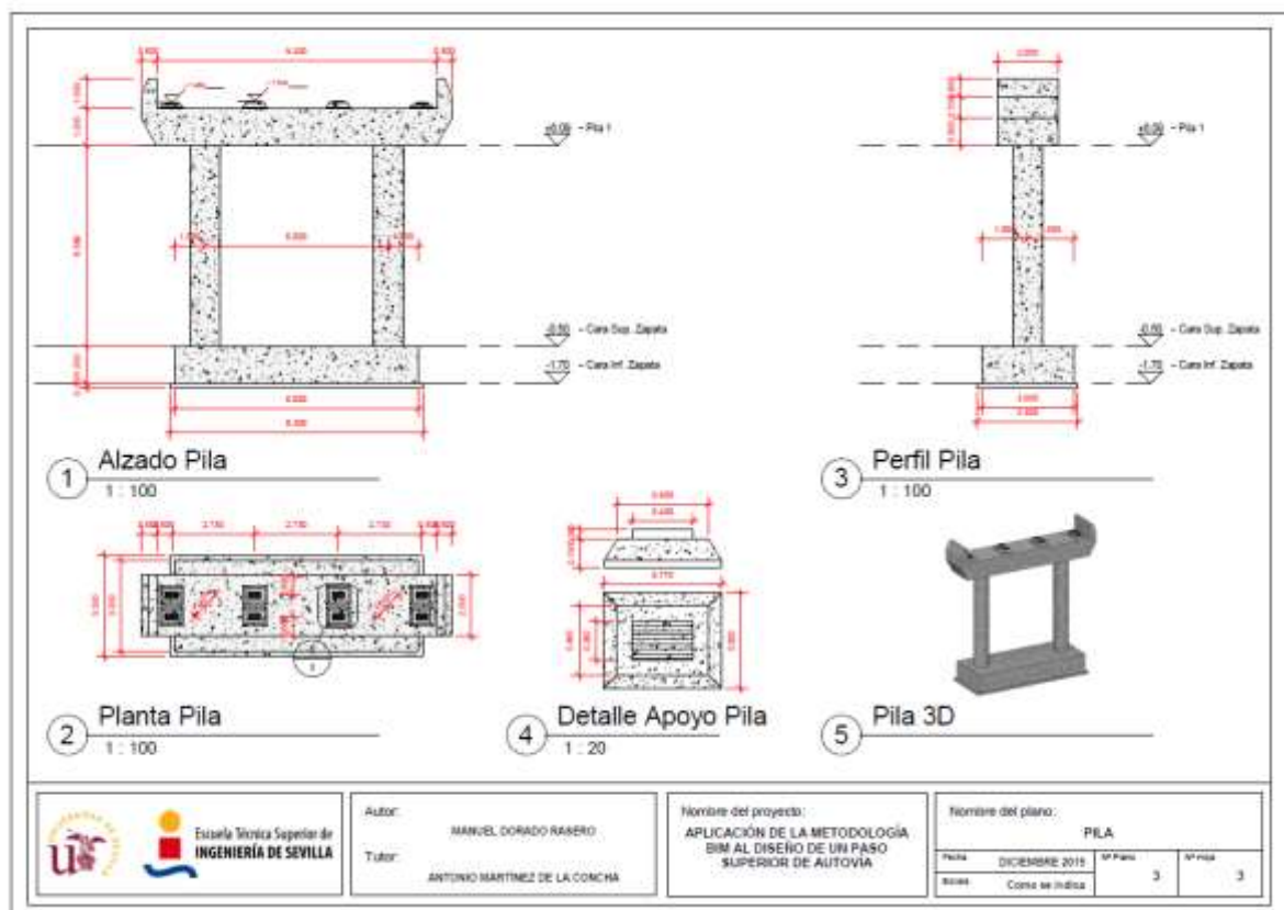
Ilustración 8.45. Ejemplo de plano realizado con Revit®. Definición geométrica de pilas. Fuente. El. prop.
