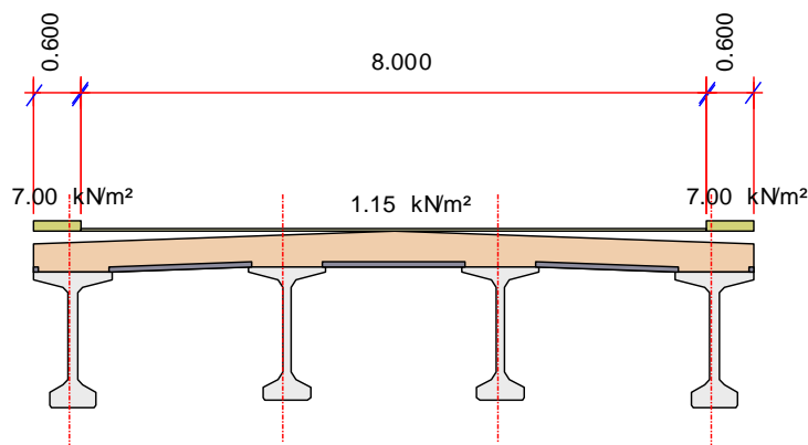
Ilustración 6.7 Acciones Permanentes sobre la superestructura. Fuente: El. prop.
