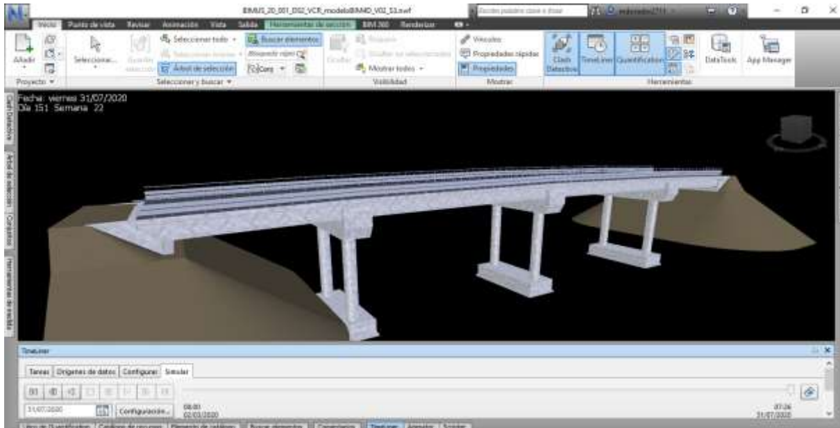
Ilustración 9.22 Apariencia final del Modelo BIM 4D. Fuente: El. prop.
