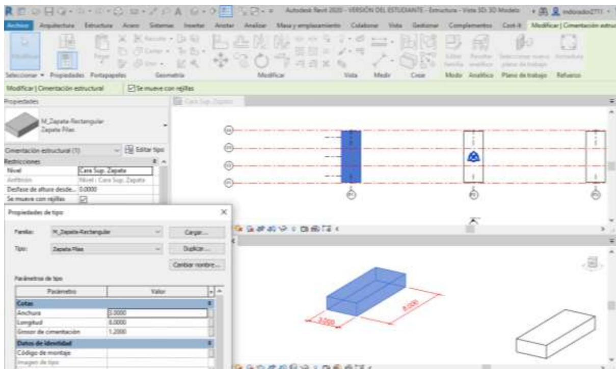
Ilustración 8.9 Introducción y Edición de zapatas en el Modelo 3D. Fuente: El. prop.
