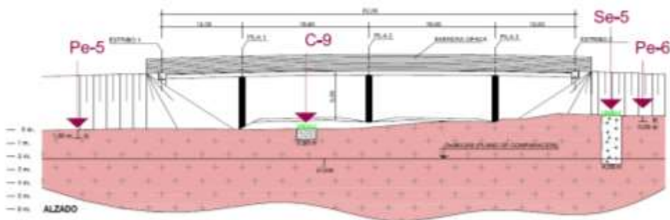
Ilustración 6.6. Perfil estratigráfico del emplazamiento. Fuente: Proyecto Original
