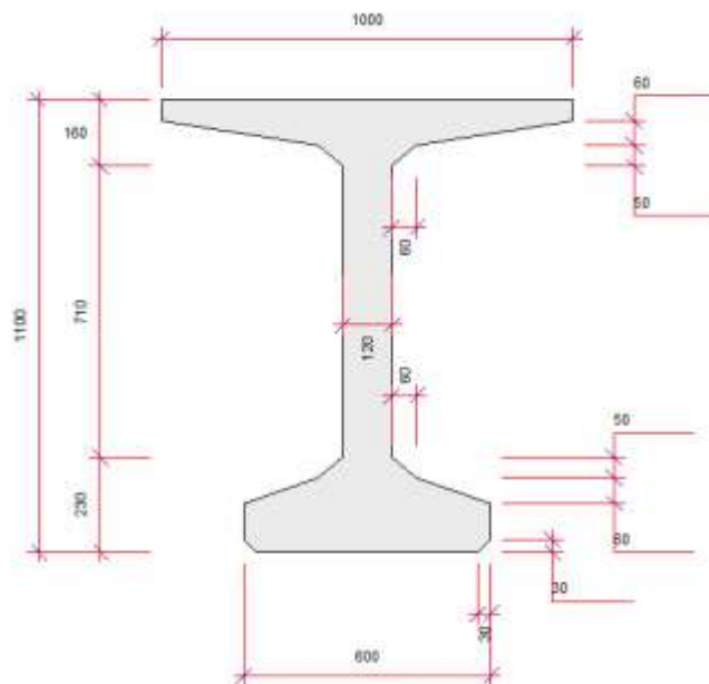
Ilustración 7.2 Sección de las vigas. Cotas en mm. Fuente: El. prop.
