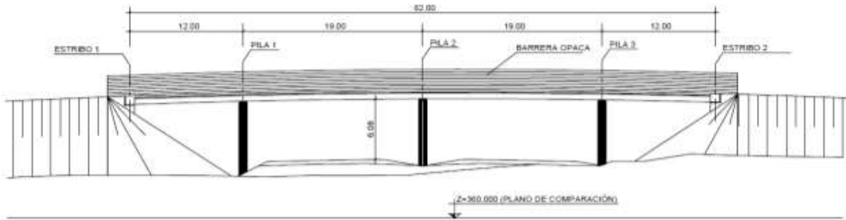
Ilustración 6.1. Alzado del Paso Superior proyectado. Fuente: Proyecto Original
