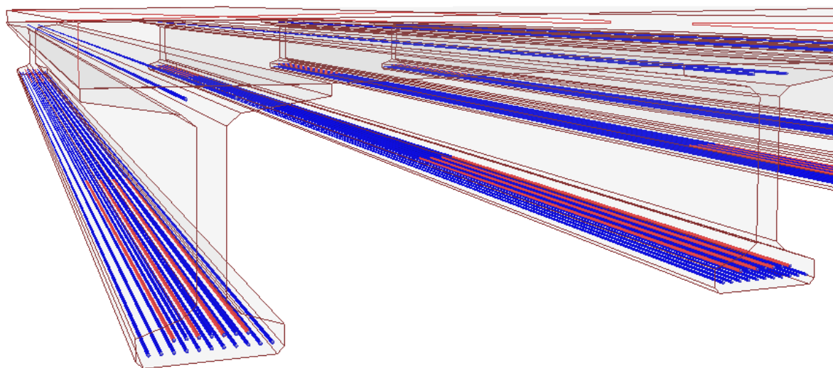
Ilustración 7.13 Vista esquemática de la armadura activa en el Tablero 2. Fuente: El. prop.
