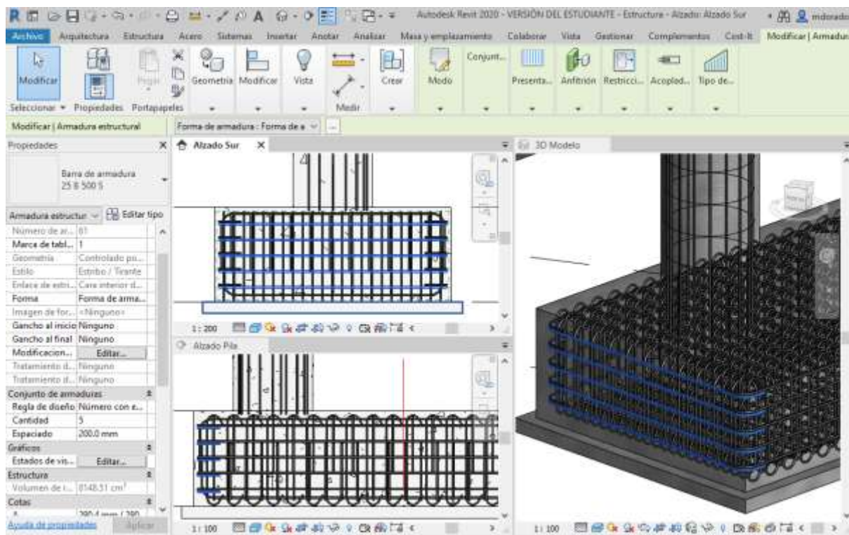
Ilustración 8.33 Introducción y edición de armaduras en el Modelo 3D. Fuente: El. prop.
