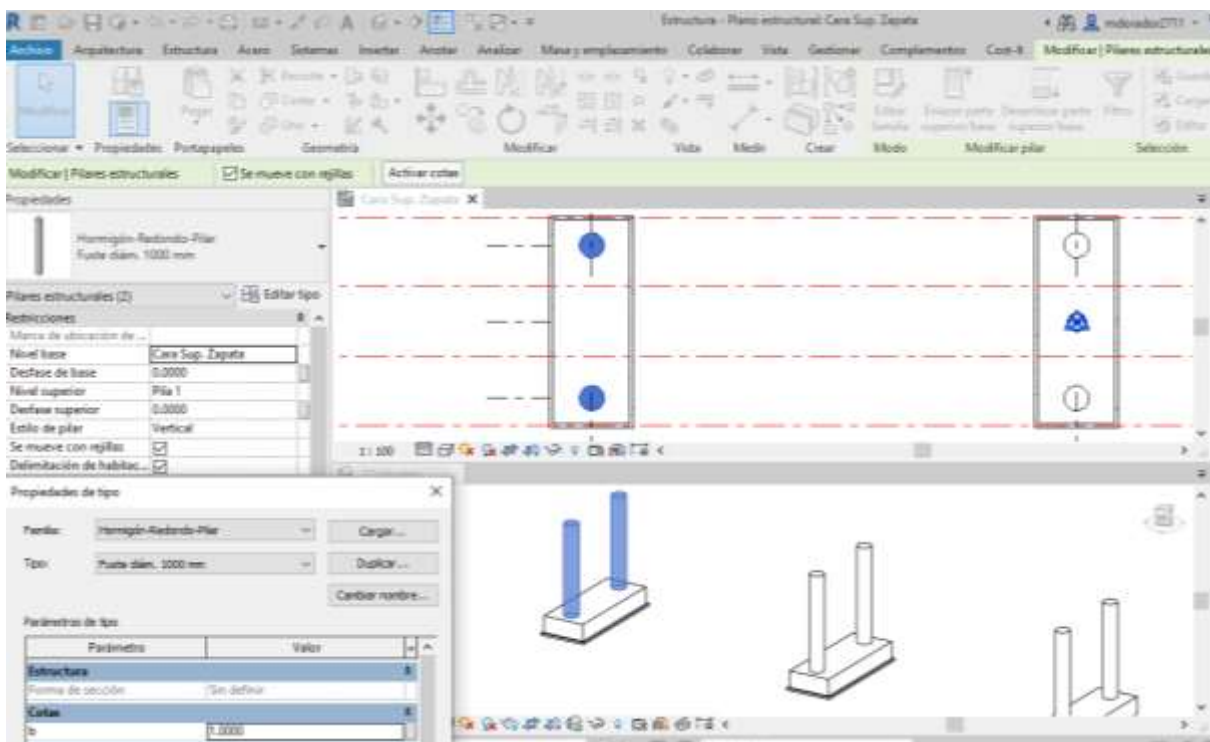
Ilustración 8.11 Introducción y edición de fustes en el Modelo 3D. Fuente: El. prop.
