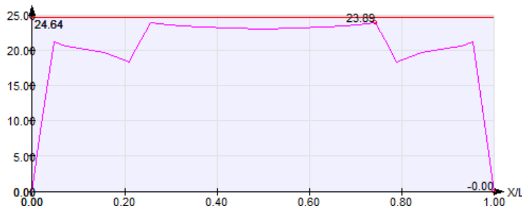
Figura 7.4 Tensiones en la fibra inferior de la Viga 2 (MPa) con 5 cordones envainados. Fuente: El. prop.
