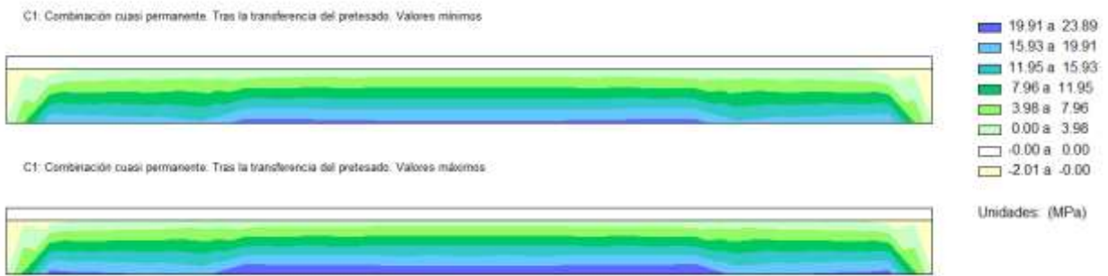
Ilustración 7.11 Valores mínimos y máximos de las tensiones en la Viga 2 para la combinación cuasi-permanente tras la transferencia de pretensado. Fuente: El. prop.
