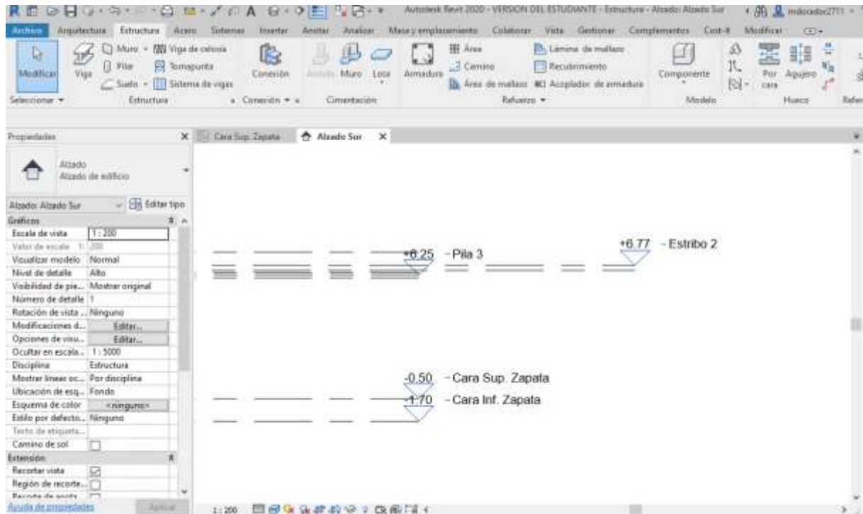
Ilustración 8.6 Definición de alturas de la estructura mediante Niveles. Fuente: El. prop..
