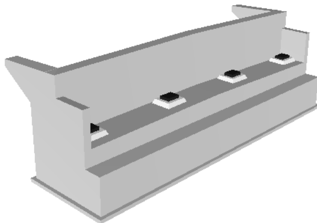
Ilustración 7.15 Vista en 3D de la tipología de estribo empleada. Fuente: El. prop.
