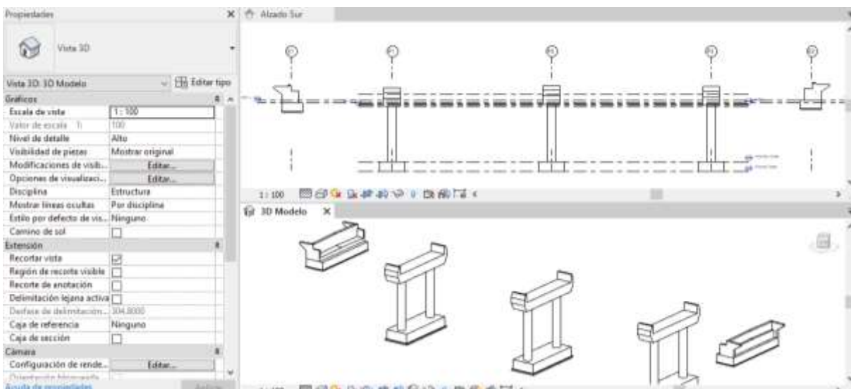
Ilustración 8.21 Pilas y Estribos del Modelo 3D. Fuente: El. prop.
