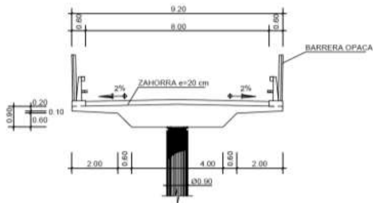
Ilustración 6.2. Sección transversal del tablero del Paso Superior proyectado. Fuente: Proyecto Original
