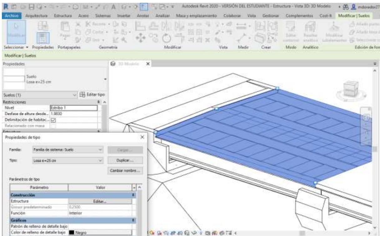
Ilustración 8.27 Introducción y edición de la losa en el Modelo 3D. Fuente: El. prop.
