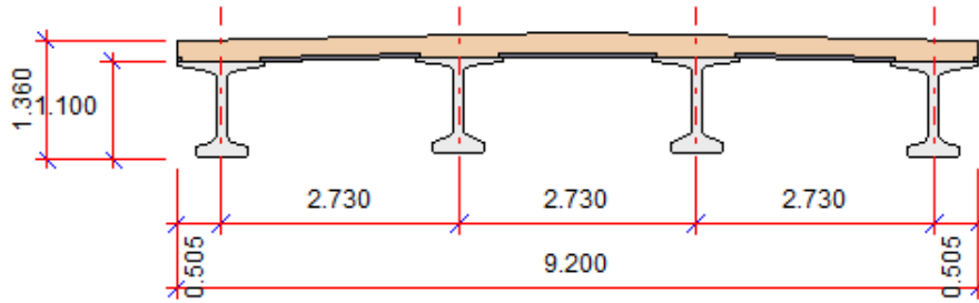
Ilustración 7.3 Vista en sección del tablero. Fuente: El. prop.
