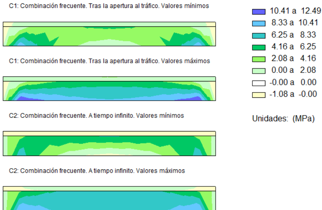
Ilustración 7.8 Valores mínimos y máximos de las tensiones en la Viga 2 para la combinación frecuente tras la apertura al tráfico y a tiempo infinito. Fuente: El. prop.
