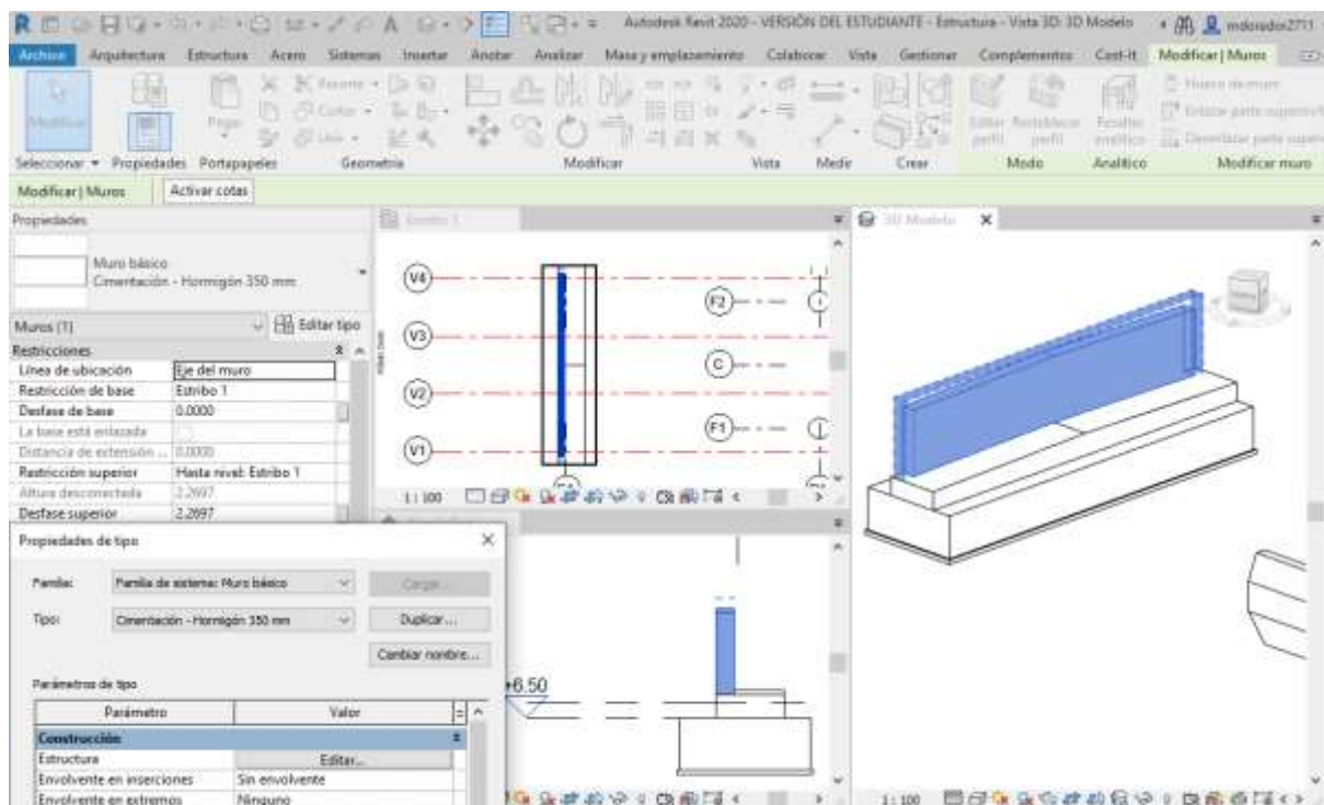
Ilustración 8.18 Introducción y edición del cargadero del Estribo 1 en el Modelo 3D. Fuente: El. prop.
