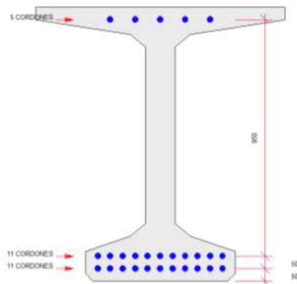
Ilustración 7.5 Armadura activa de las vigas. Fuente: El. prop.
