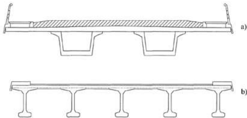
Ilustración 6.4. Tipos de vigas prefabricadas. Fuente: Manterola, Javier “Puentes I”[58]
