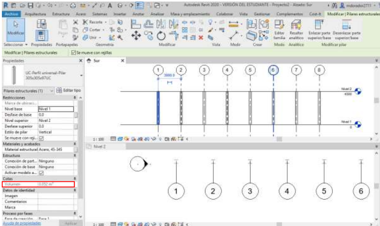
Ilustración 8.8 Edición de elementos en Revit® modificando los niveles. Fuente: El. prop.
