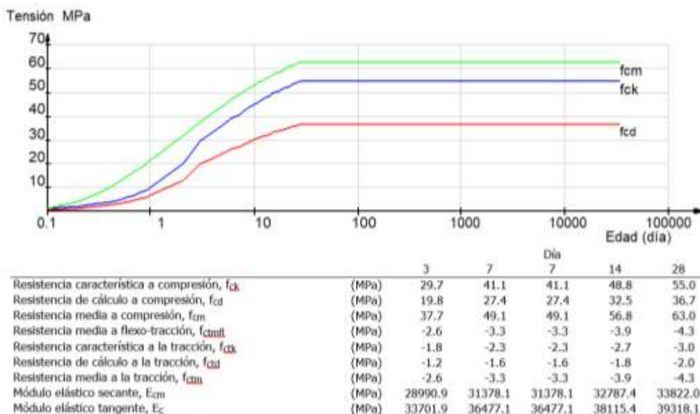
Figura 7.1 Resistencia a compresión de un hormigón HA-55. Fuente: El. prop.
