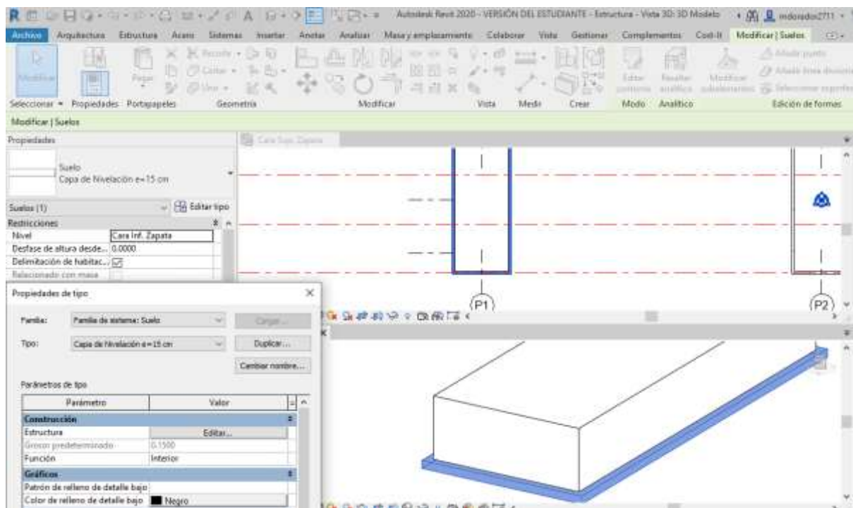
Ilustración 8.10 Introducción y edición de las capas de nivelación en el Modelo 3D. Fuente: El. prop.
