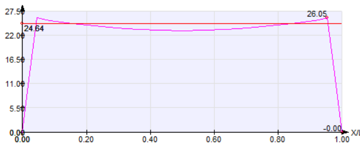
Figura 7.3 Tensiones en la fibra inferior de la Viga 2 (MPa). Fuente: El. prop.
