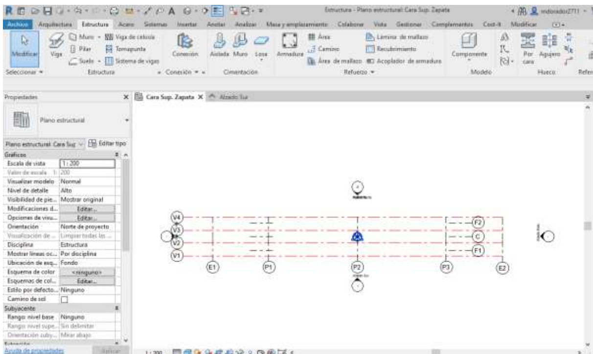
Ilustración 8.5 Definición de vanos y ejes de la estructura mediante Rejillas. Fuente: El. prop.
