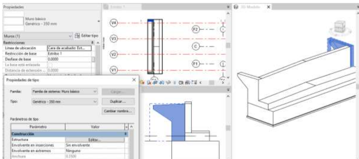
Ilustración 8.19 Introducción y edición de aletas del Estribo 1 en el Modelo 3D. Fuente: El. prop.
