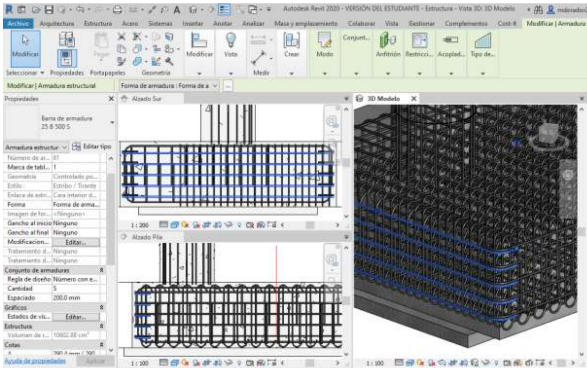
Ilustración 8.34 Modificación de armaduras en el Modelo 3D. Fuente: El. prop.
