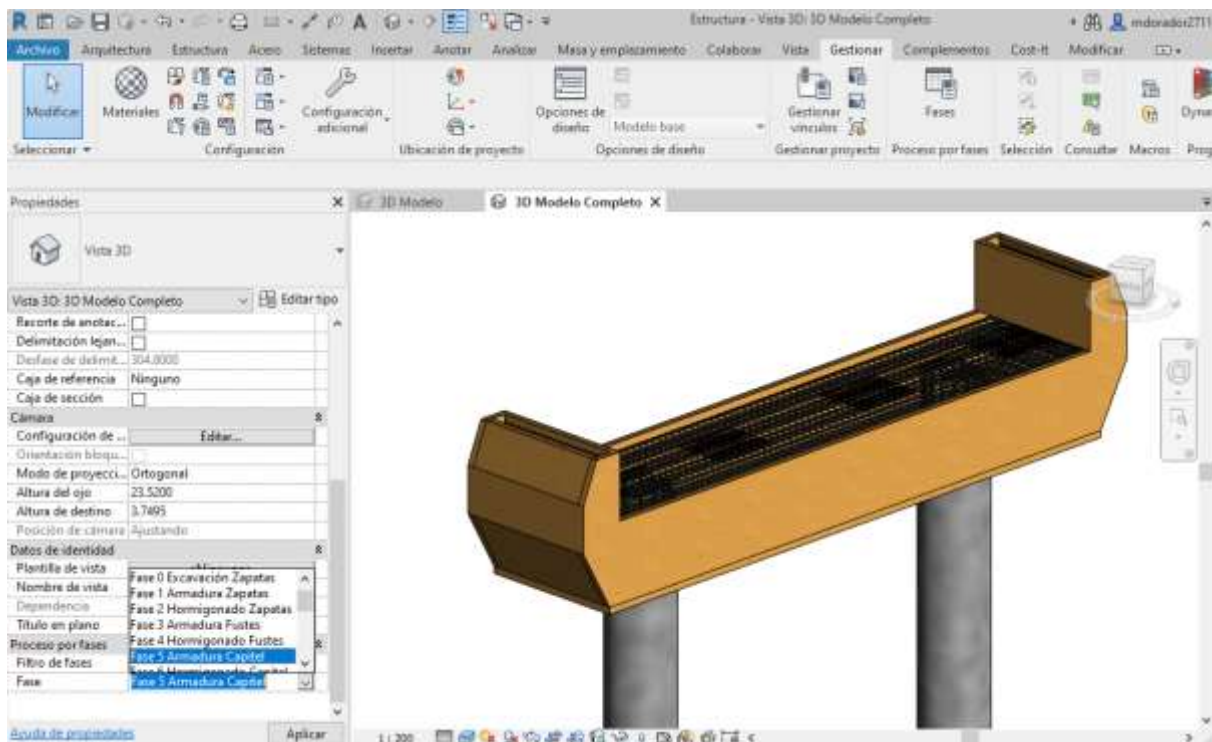
Ilustración 8.41 Simulación de fases de la construcción en el Modelo 3D. Fase 5. Fuente: El. prop.
