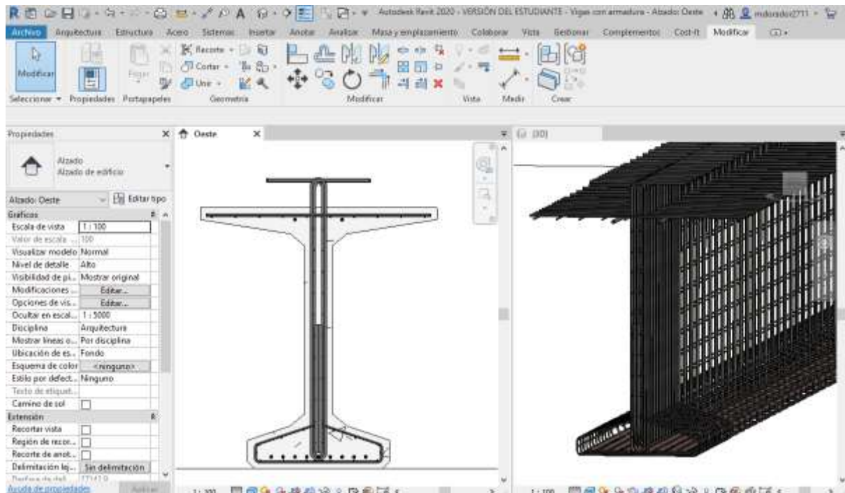
Ilustración 8.37 Introducción de armaduras en las vigas. Fuente: El. prop.
