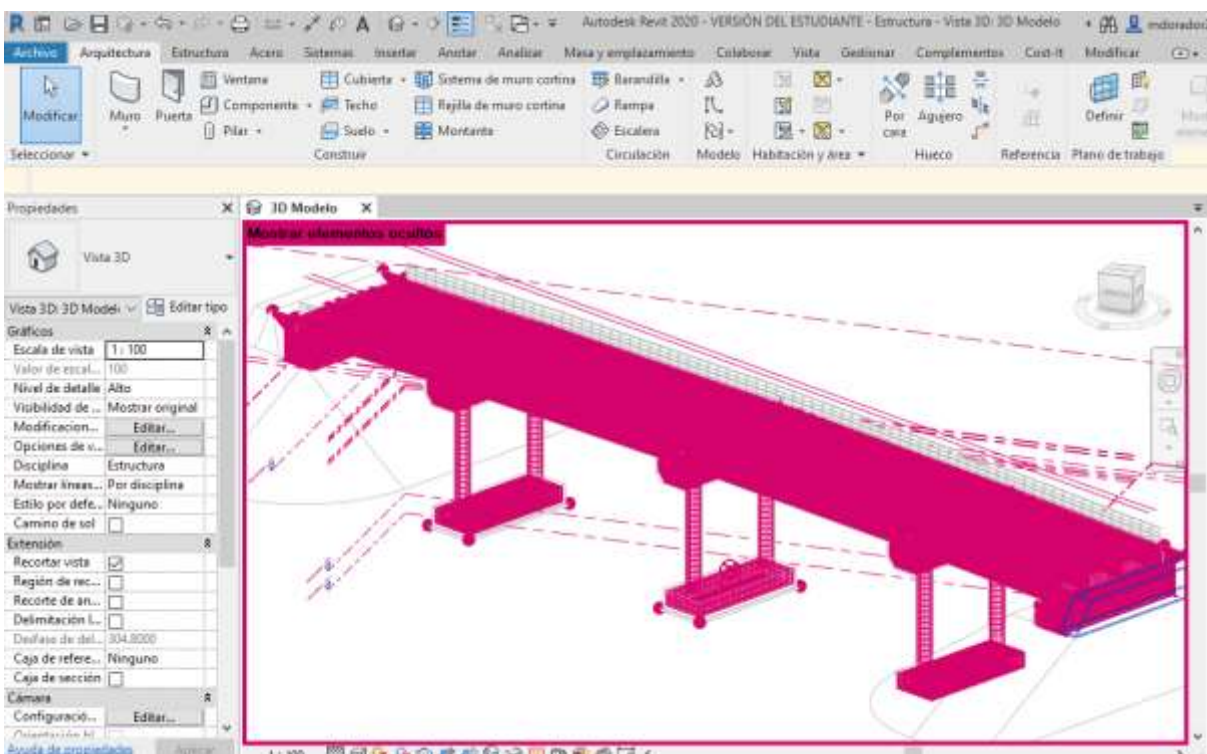
Ilustración 8.35 Armadura oculta en el Modelo 3D. Fuente: El. prop.
