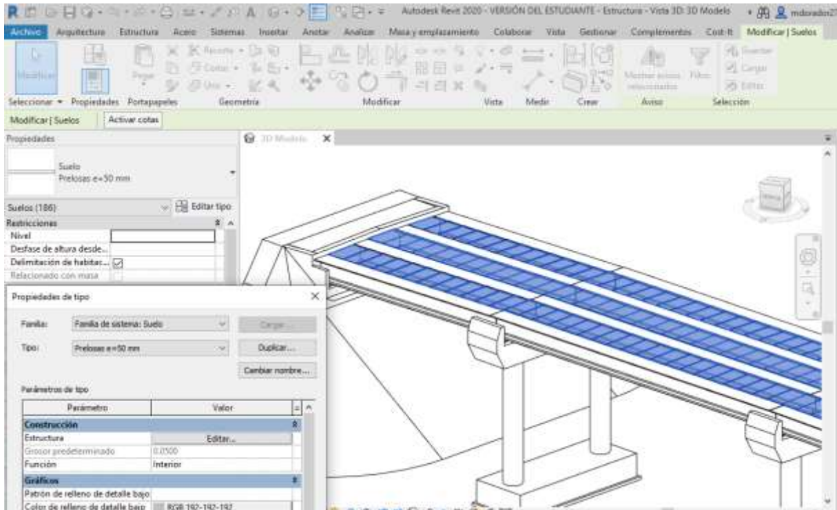
Ilustración 8.26 Introducción y edición de prelosas en el Modelo 3D. Fuente: El. prop.
