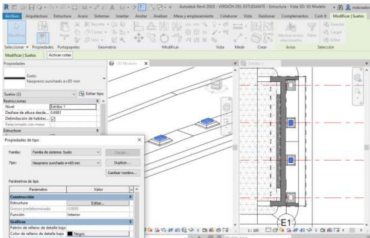
Ilustración 8.22 Introducción y edición de apoyos en el Modelo 3D. Fuente: El. prop.
