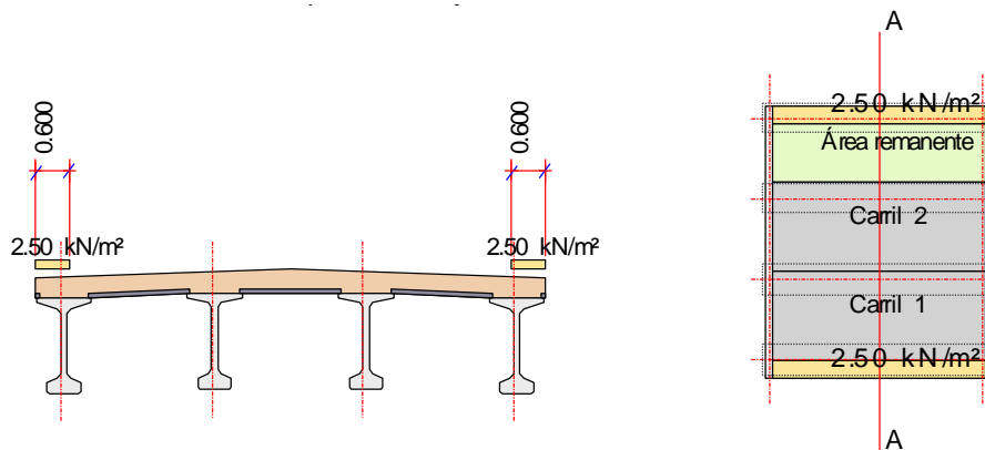
Ilustración 6.9 Acciones variables. Sección del tablero (izda.) y definición de carriles virtuales, hipótesis 2 (dcha.). Fuente: El. prop.
