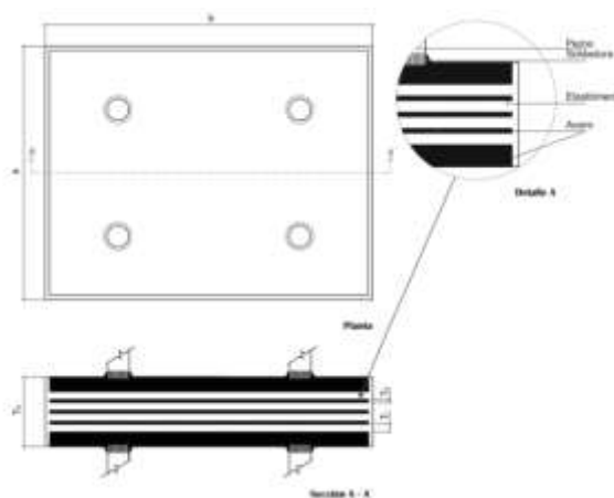
Ilustración 7.16 Sección de apoyos con anclaje mediante pernos. Fuente: El. prop.
