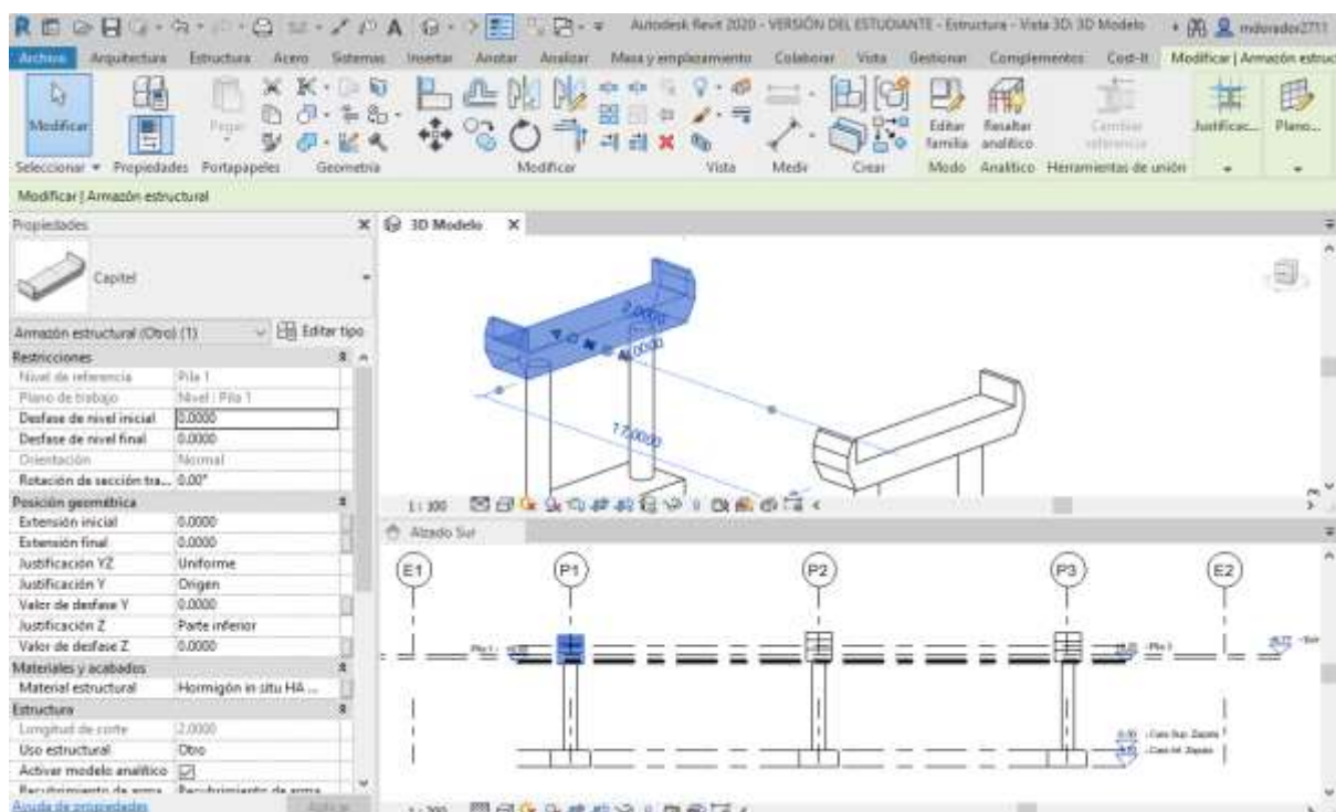
Ilustración 8.13 Introducción y edición de la viga capitel en el Modelo 3D. Fuente: El. prop.
