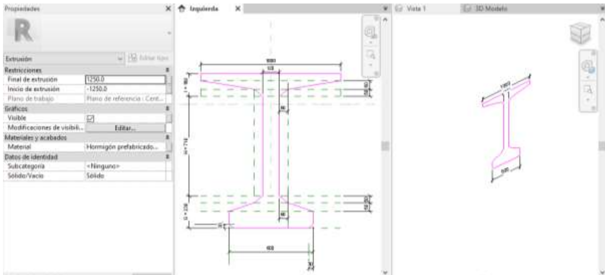
Ilustración 8.23 Edición de la sección de la viga con el editor de familias. Fuente: El. prop.
