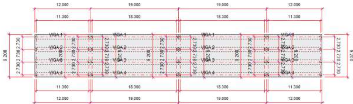
Ilustración 7.4 Vista en planta del tablero. Fuente: El. prop.
