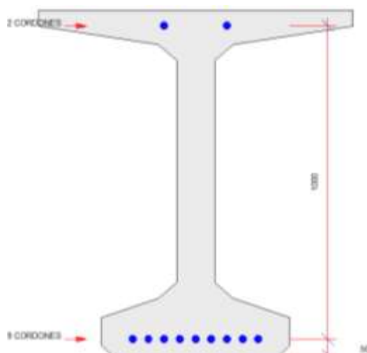
Ilustración 7.6 Armadura activa de las vigas de los tableros 1 y 4. Fuente: El. prop.
