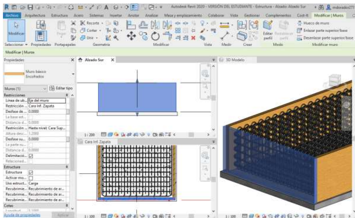
Ilustración 8.38 Introducción y edición de encofrados en el Modelo 3D. Fuente: El. prop.
