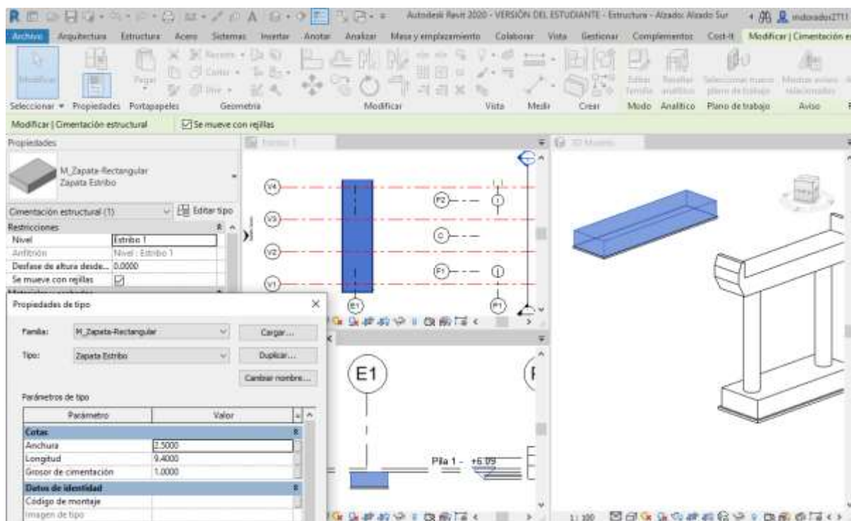
Ilustración 8.15 Introducción y edición de la zapata del Estribo 1 en el Modelo 3D. Fuente: El. prop.
