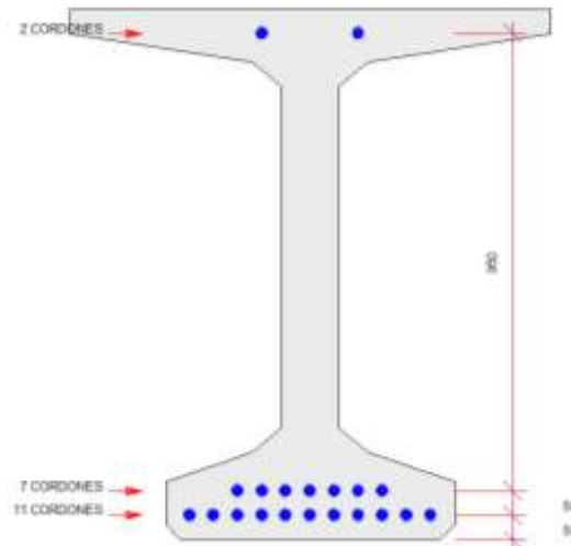
Ilustración 7.10 Armadura activa de las vigas de los tableros 2 y 3. Fuente: El. prop.
