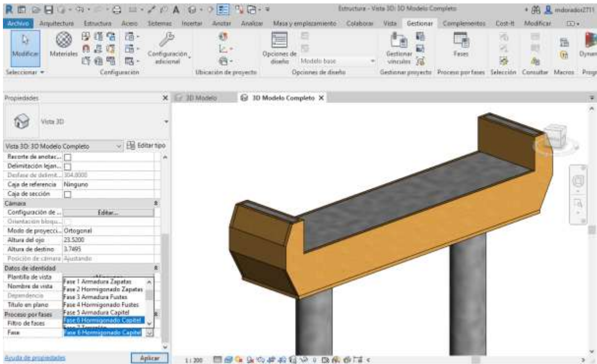
Ilustración 8.42 Simulación de fases de la construcción en el Modelo 3D. Fase 6. Fuente: El. prop.
