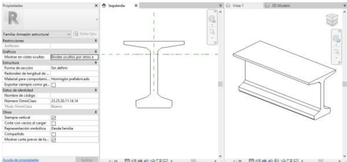
Ilustración 8.24 Apariencia final de la viga creada. Fuente: El. prop.
