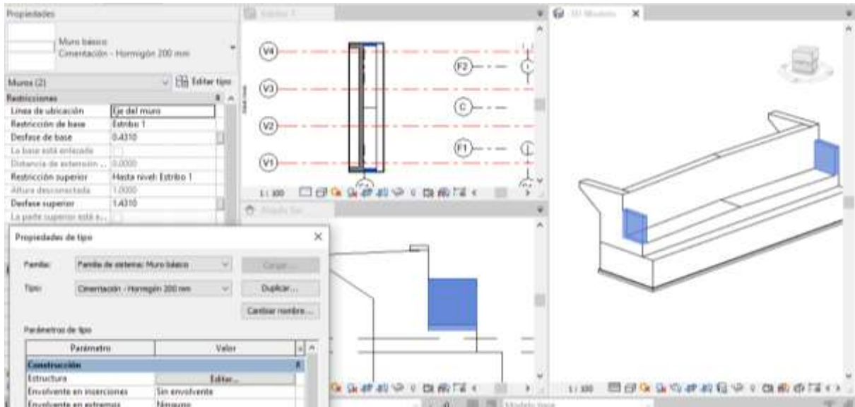
Ilustración 8.20 Introducción y edición de los muretes laterales del Estribo 1 en el Modelo 3D. Fuente: El. prop.
