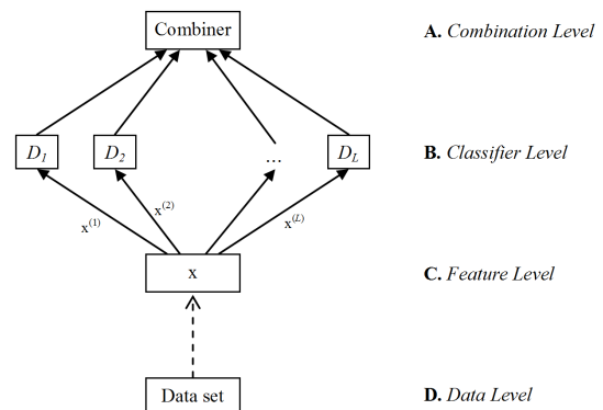
Figura 2: Enfoques para la combinación de clasificadores.
