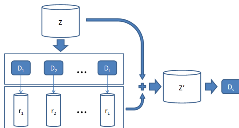
Figura 3: Esquema general del Stacking
