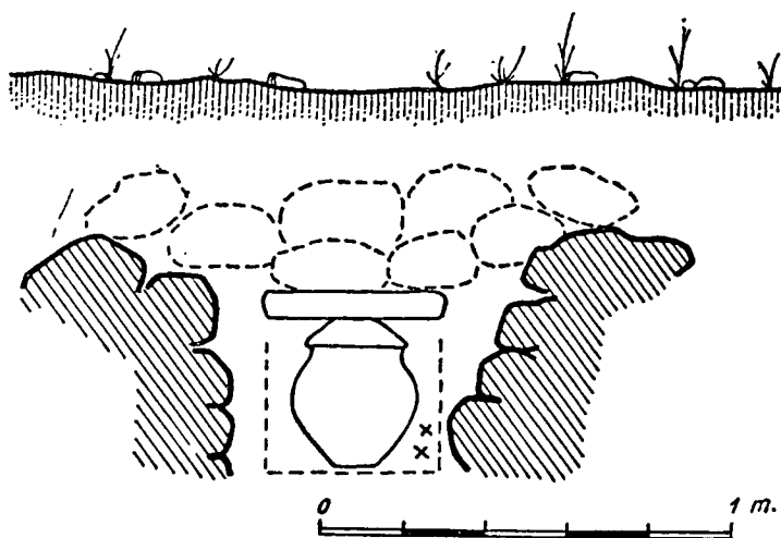
Fig. 2.—Tumba núm. 5 de la necrópolis fenicia del Cortijo de las Sombras (Frigiliana, Málaga), según Arribas y Wilkins.
