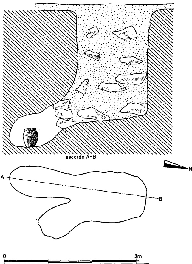
Fig. 6.—Planta y perfil de la T. núm. 15. Necrópolis de Almuñécar (Granada). S. M. Pellicer.
