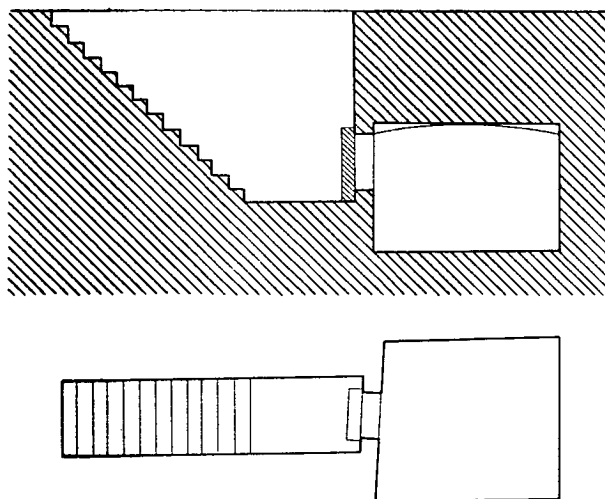
Fig. 8.—Tumba de cámara con escalera. Necrópolis de Jbel-Mlezza (Túnez). S. Gobert y Cintas.
