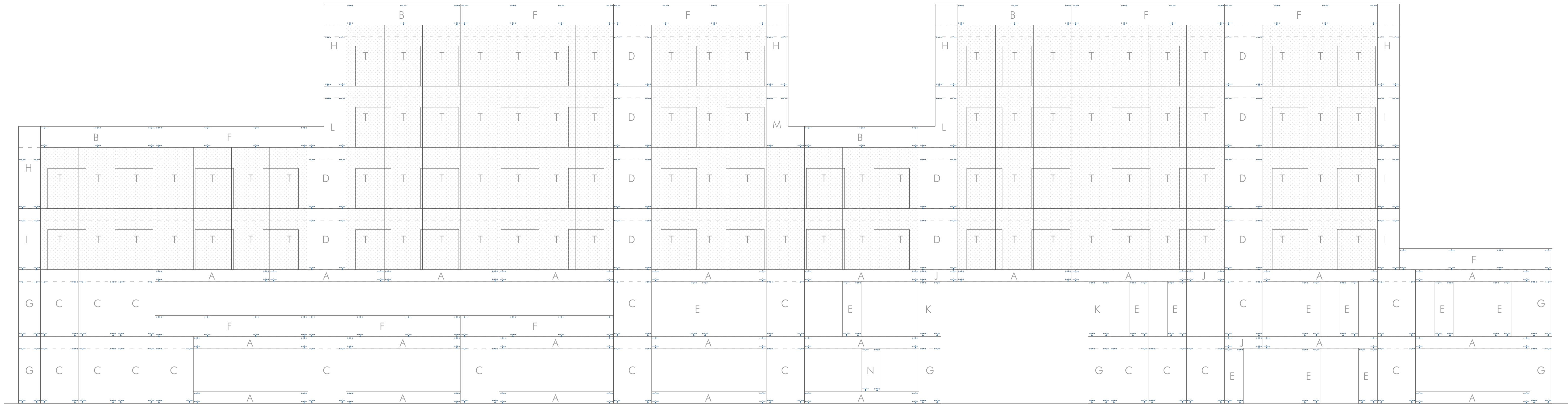
Despiece Fachada Oeste 1:100 --- Línea de Forjado --- Anclaje de apoyo ▲ Anclaje de apoyo y carga
