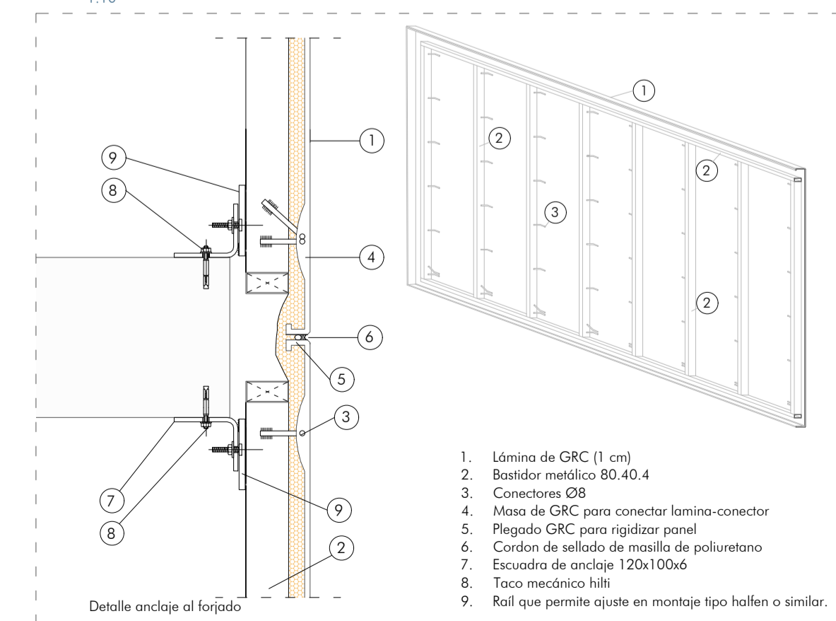
Panel Stud Frame 1:10
